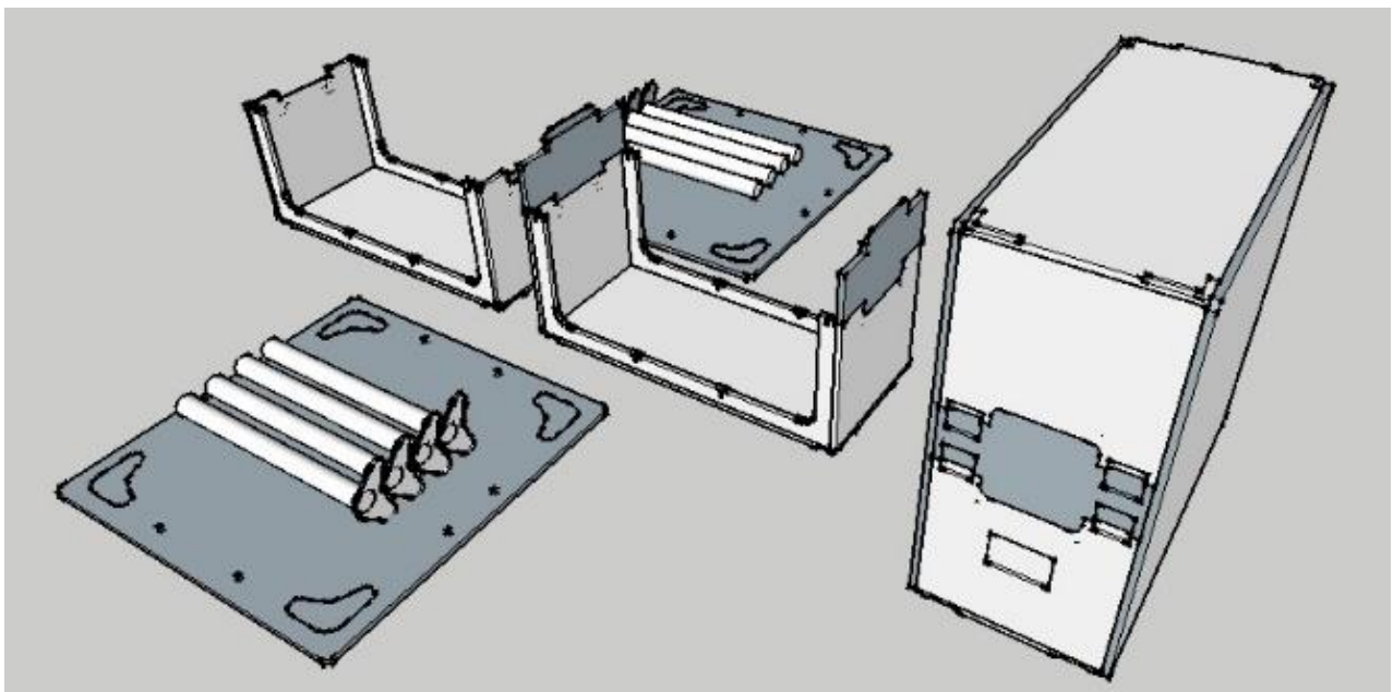
A gauche, les composants du kit de base de la box ariab (2 plateaux et leurs 8 pieds, 2 bancs et 2 pièces d'assemblage), et à droite la box ariab assemblée
